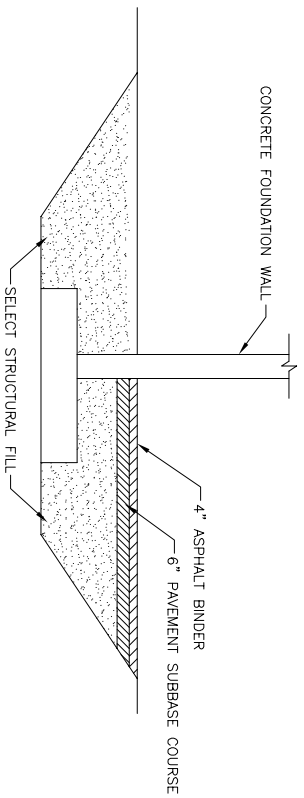
FOUNDATION BACKFILL SECTION SCALE: N.T.S.
