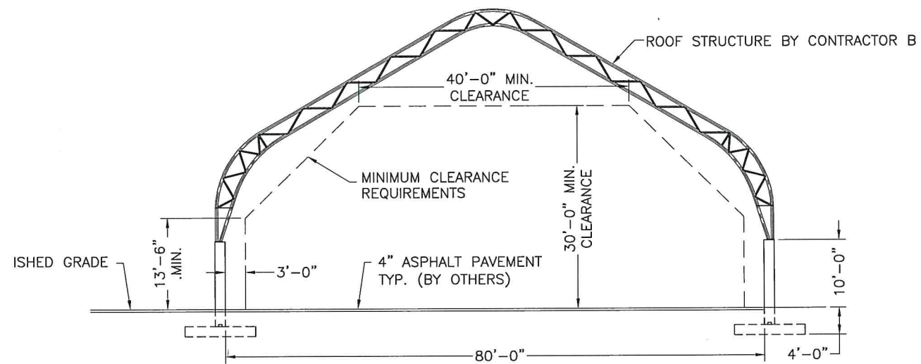
ELEVATION
